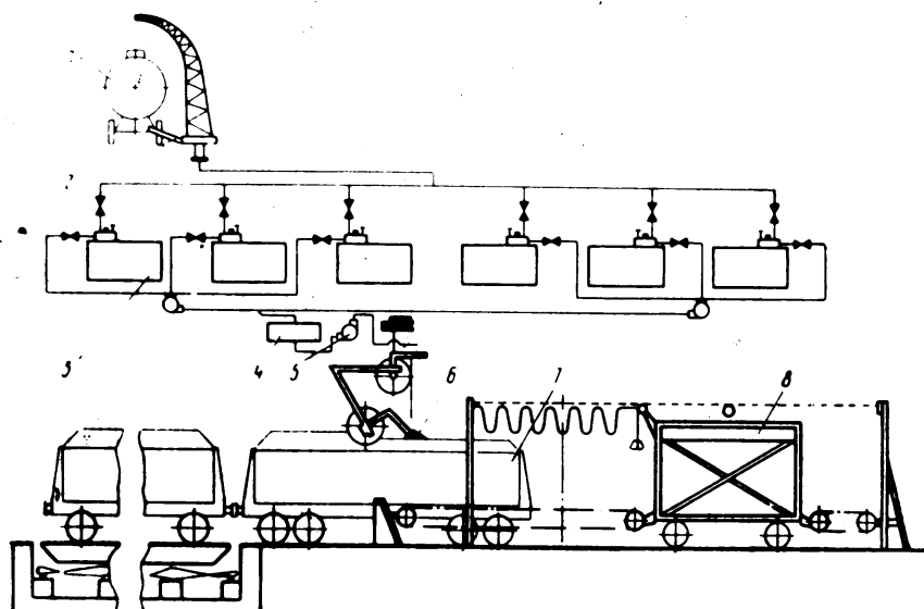
Рис. 16.1. Схема нанесення захисної плівки на поверхню ущільненого вугілля
