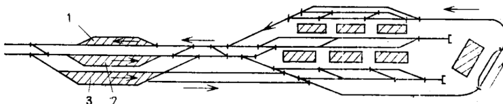
Рис. 13.3. Поліпшена тупикова схема внутрішньозаводських колій: 1 – парк відправлення; 2 – парк прибуття; 3 – сортувальний парк
