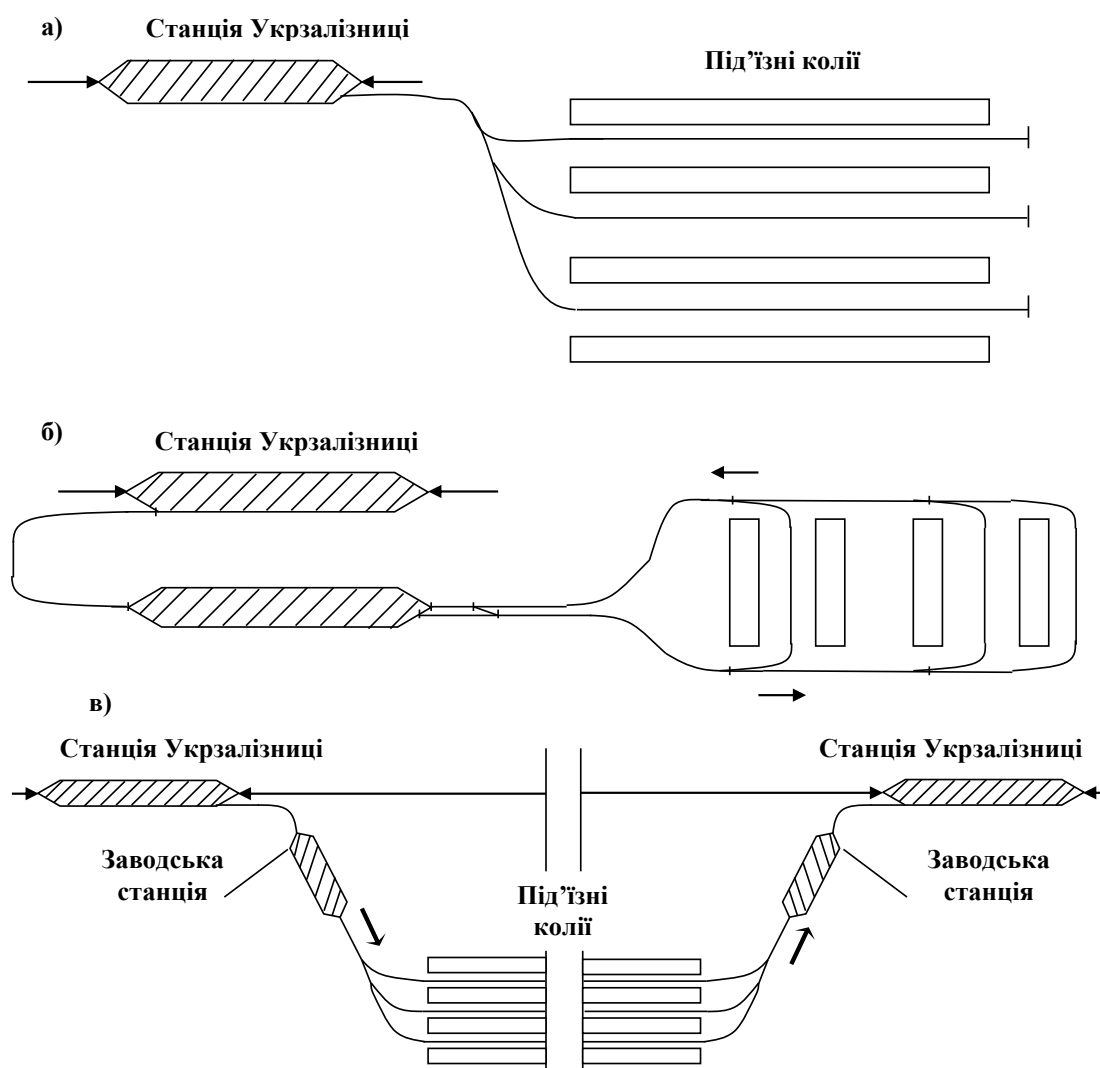
Рис. 13.1. Варіанти розвитку під'їзних колій
