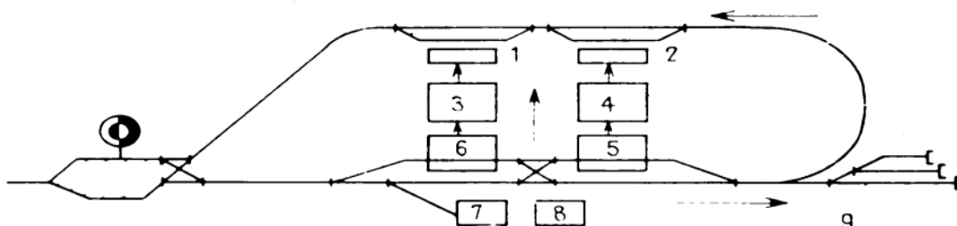
Рис. 13.4. Кільцева схема залізничних колій: 1–2 – склади готової продукції; 3–4 – складальні цехи; 5 – ковальський цех; 6 – ливарний цех; 7 – склад вугілля; 8 – ТЕЦ; 9 – обробний цех
