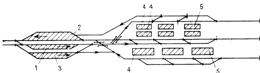
Рис. 13.2. Тупикова схема внутрішньозаводських колій: 1 – парк прибуття; 2 – парк відправлення; 3 – сортувальний парк; 4 – склади сировини; 5 – склади готової продукції
