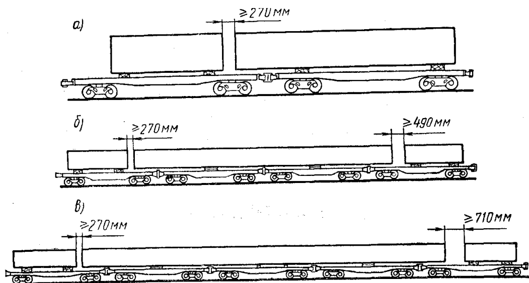
Рис. 20.3. Відстані між вантажами на платформах прикриття: а – розміщення довгомірних вантажів на суміжних платформах; б – розміщення довгомірних вантажів на двох вагонах за наявності звисання; в – розміщення довгомірних вантажів на суміжних платформах за наявності проміжної платформи прикриття
