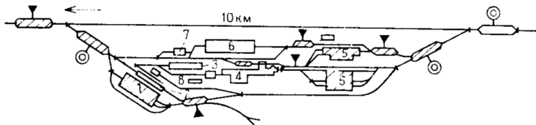
Рис. 13.5. Двостороння схема колій металургійного заводу з двома примиканнями до лінії загального користування: 1 – коксохімічний цех; 2 – доменний цех; 3 – мартенівський цех; 4 – прокатний цех; 5 – трубопрокатний цех; 6 – допоміжні і ремонтні цехи; 7 – тягове господарство; 8 – вугільний склад і ТЕЦ
