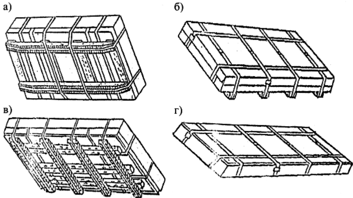
Рис. 20.6. Розміщення та кріплення листового металлу: а – на санчатах; б – на поперечних брусках; в – на піддонах; г – без дерев'яних реквізитів
