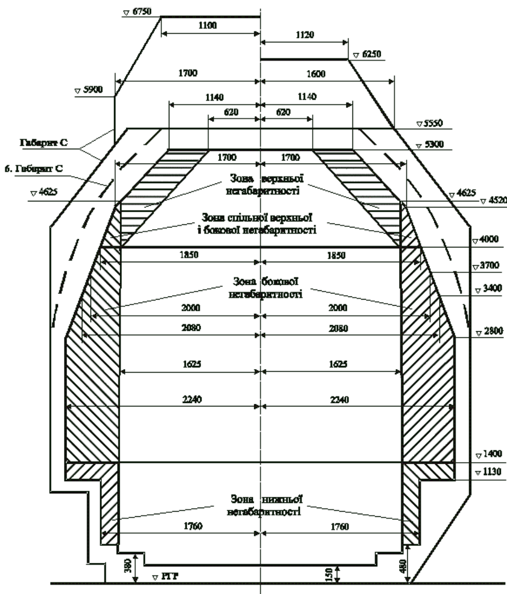
Рис. 20.2. Зони негабаритності вантажу
