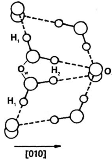
Рисунок 3 - Конфигурация водородных мостиковых связей в \text{CaSO}_4 \cdot 2\text{H}_2\text{O} [8]
