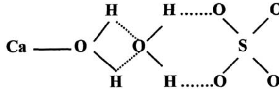
Рисунок 4 - Водородная связь в структуре двухводного гипса [9]
