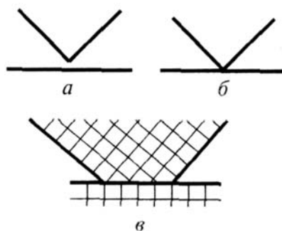
Рисунок 1 - Контакты между частицами: а и б – коагуляционные, в - фазовый
