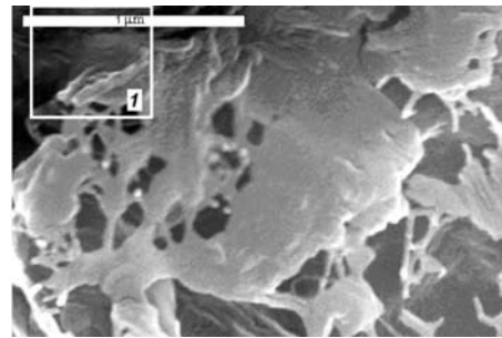
Рисунок 6 - ЭМС гидросиликатов кальция
