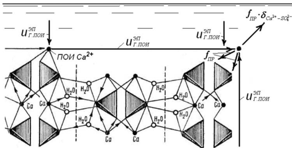
Рисунок 12 - Схема действия давления от энергии электроповерхностной гидратации ПОИ
