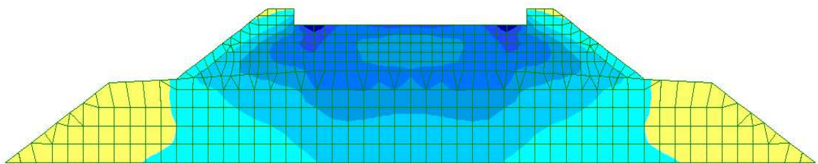
Рис. 1. Напружений стан баластної призми без посилення
